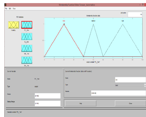
Fig 9.FD fan output
