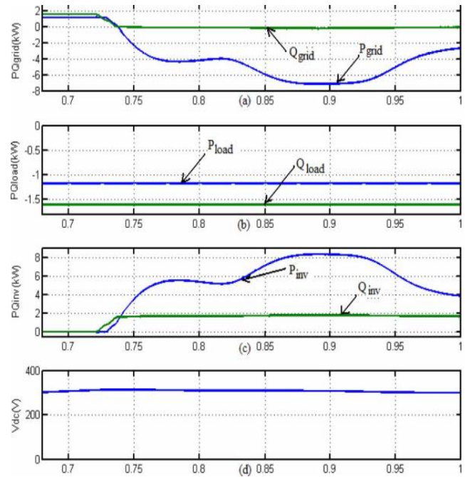
Fig. (5) Simulation results: (a) PQ-Grid, (b) PQ-Load, (c) PQ-Inverter, (d) dc-link voltage
