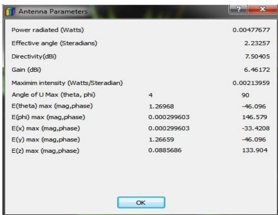
Fig. 7: Antenna Parameters
