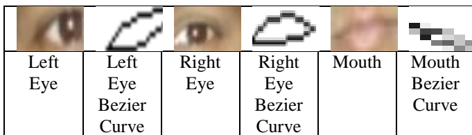
Fig 3.4.1 Bezier Curve
